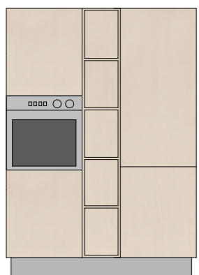
PROSPETTO COLONNE
